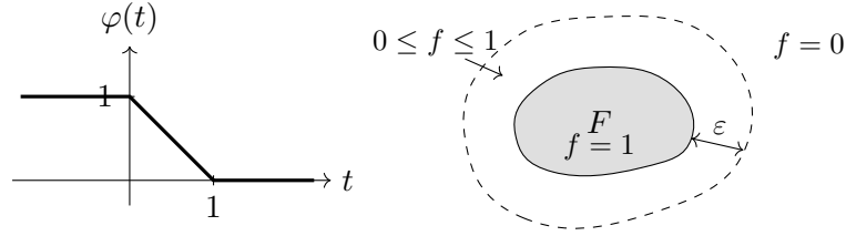
Abbildungung 2.2.: Links: die Funktion \varphi aus (2.2). Rechts: Die Funktion f = \varphi(d(\cdot, F)/\varepsilon) ist gleich 1 auf F , gleich 0 außerhalb der \varepsilon -Umgebung von F (gestrichelt) und fällt dazwischen linear im Abstand zu F ab.
