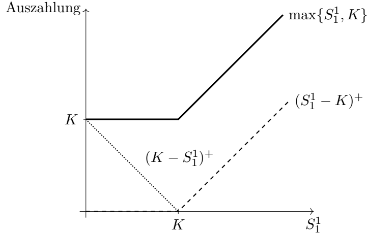
Abbildung 8.1.: Auszahlungen von Call und Put zum Strike K . Portfolio I liefert (S_1^1 - K)^+ + K , Portfolio II liefert (K - S_1^1)^+ + S_1^1 ; beide stimmen mit \max\{S_1^1, K\} überein.
