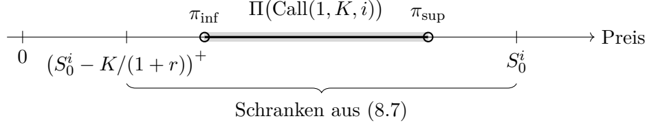
Abbildungung 8.4.: Die Menge der arbitragefreien Preise eines Calls ist ein Intervall innerhalb der Schranken aus (8.7). Ist der Call nicht replizierbar, so ist das Intervall nach Satz 8.26 offen.
