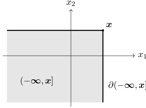
Abbildung 1.1.: Der Quadrant (-\infty, \mathbf{x}] für k = 2 ; der Rand ist fett eingezeichnet.
