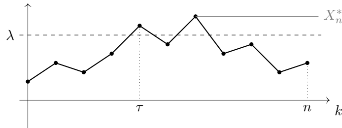
Abbildung 7.1.: Zum Beweis von Lemma 7.1: Überschreitet der Pfad bis zur Zeit n das Niveau \lambda , so stoppt \tau beim ersten Überschreiten mit X_\tau \geq \lambda ; andernfalls ist \tau = n .
