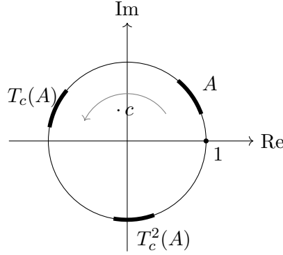
Abbildung 4.1.: Zum Beweis von Satz 4.9 für c = e^{2\pi i/3} , also c^3 = 1 : Die Vereinigung B = A \cup T_c(A) \cup T_c^2(A) der gedrehten Kopien eines kleinen Bogens A ist T_c -invariant, hat aber Maß in (0, 1) .
