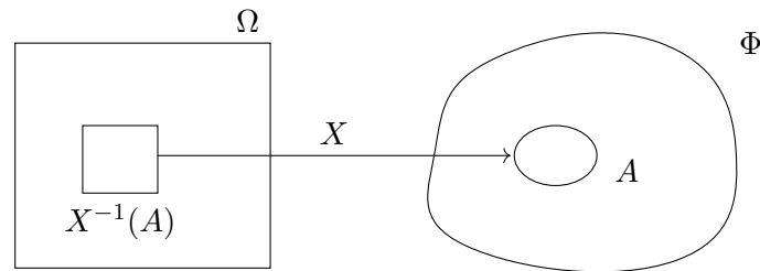
Abbildung 1.: Urbild einer Menge A \in \mathcal{G} unter einer Zufallsvariablen X .
