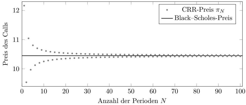
Abbildungung 9.3.: CRR-Preise eines europäischen Calls in Abhängigkeit von der Anzahl N der Perioden und der Grenzwert (9.8), für S_0^1 = K = 100 , T = 1 , \rho = 0,05 und \sigma = 0,2 ; der Black-Scholes-Preis beträgt hier etwa 10,45.
