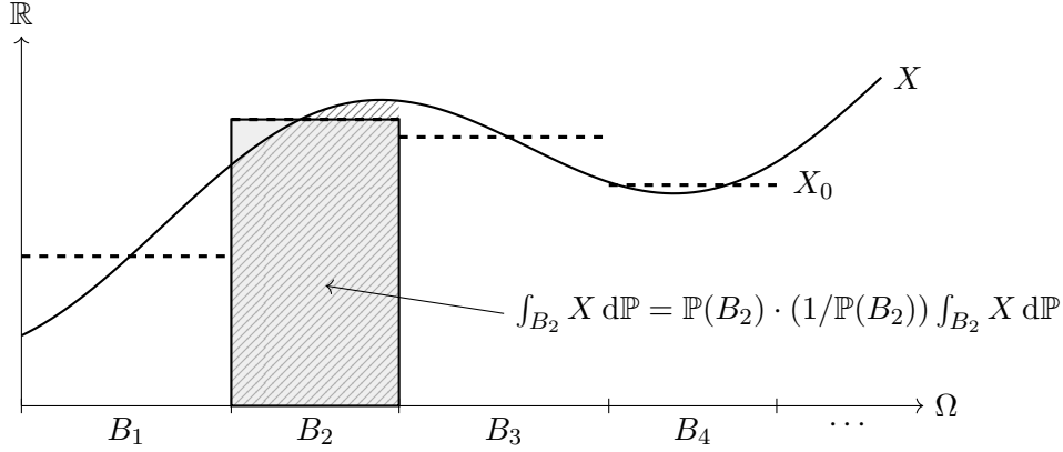
Abbildung 5.1.: Die Zufallsvariable X_0 aus (5.1) (gestrichelt) ist auf jeder Menge B_i der Partition konstant gleich dem Mittelwert von X auf B_i . Die schraffierte Fläche unter X über B_2 und das fett umrandete Rechteck über B_2 mit der Höhe des Mittelwerts haben denselben Inhalt.
