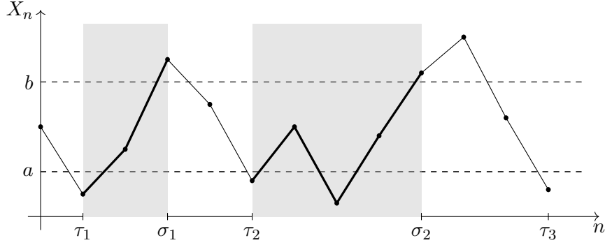
Abbildung 7.2.: Ein Pfad von X mit den Stoppzeiten \tau_k und \sigma_k . Die beiden Aufkreuzungen über [a, b] sind fett gezeichnet; grau unterlegt sind die Zeiten m \in \{\tau_k + 1, \dots, \sigma_k\} , zu denen die Strategie H aus dem Beweis von Lemma 7.3 investiert ist. Hier gilt U_{12}^{a,b} = 2 .
