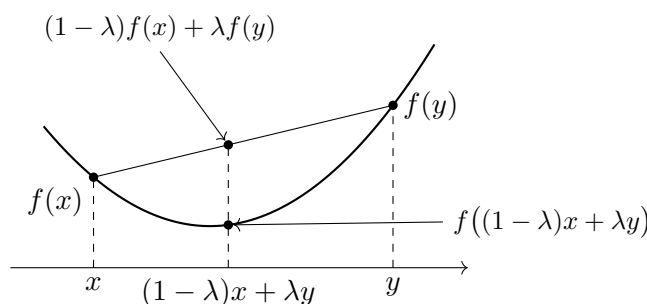
Abbildung 3.1.: Eine konvexe Funktion: Die Sehne zwischen (x, f(x)) und (y, f(y)) liegt oberhalb des Graphen.
