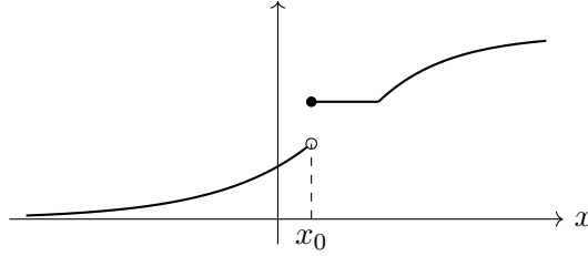
Abbildung 2.7.: Eine maßdefinierende Funktion mit einem Sprung in x_0 ; dort ist sie rechtsseitig stetig, und das zugehörige Maß \mu_F hat ein Atom in x_0 .
