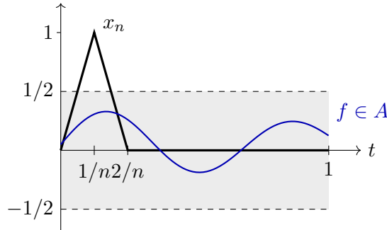
Abbildung 2.6.: Die Zeltfunktion x_n aus Beispiel 2.32 und die Menge A der Funktionen, deren Graph im grauen Streifen liegt. Für jedes feste t > 0 gilt x_n(t) = 0 für große n , aber x_n \notin A .
