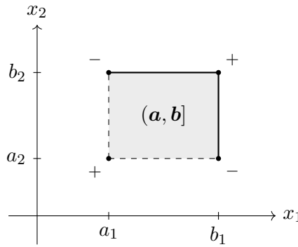
Abbildung 2.5.: Der Quader (\mathbf{a}, \mathbf{b}] für k = 2 . Seine Wahrscheinlichkeit ergibt sich aus den Werten der Verteilungsfunktion an den vier Ecken mit den eingezeichneten Vorzeichen.
