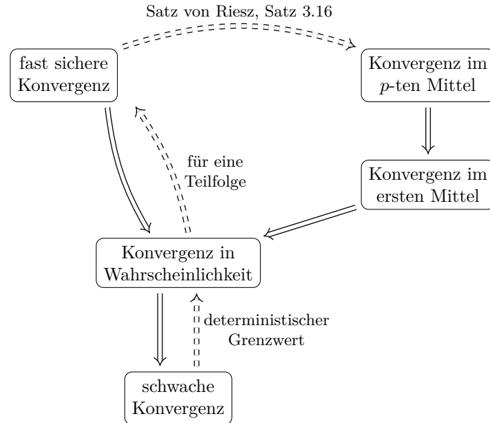
Abbildung 3.3.: Zusammenhang der Konvergenzarten für Zufallsvariablen auf einem Wahrscheinlichkeitsraum. Gestrichelte Pfeile gelten nur unter Zusatzbedingungen.
