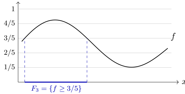
Abbildung 2.4.: Approximation von \int f d\mathbb{P}_n durch die Niveaumengen F_i = \{f \geq i/k\} im Beweis von Satz 2.23, hier für k = 5 . Auf \{(i-1)/k \leq f < i/k\} = F_{i-1} \setminus F_i liegt f zwischen (i-1)/k und i/k .
