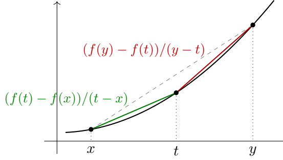
Abbildung 3.2.: Die Steigungsbedingung (3.2): Die linke (grüne) Sekante ist flacher als die rechte (rote). Die gestrichelte Sekante von x nach y liegt mit ihrer Steigung dazwischen.
