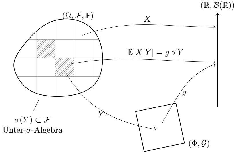
Abbildung 5.3.: Die bedingte Erwartung \mathbb{E}[X|Y] ist \sigma(Y) -messbar und faktorisiert daher als g \circ Y ; sie hängt von \omega nur über die Beobachtung Y(\omega) ab.
