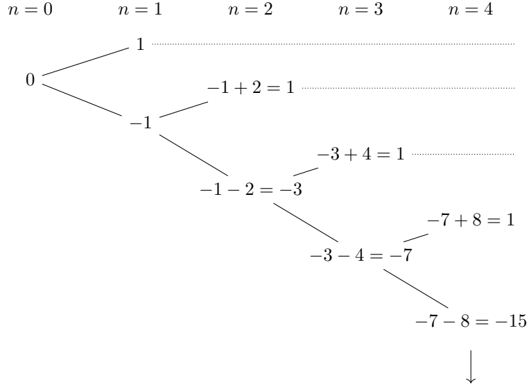
Abbildung 7.3.: Mögliche Werte von S_n im Petersburger Spiel. Nach dem ersten Gewinn bleibt S_n = 1 ; der Pfad, auf dem nur verloren wird, hat Wahrscheinlichkeit 2^{-n} und den Wert 1 - 2^n .
