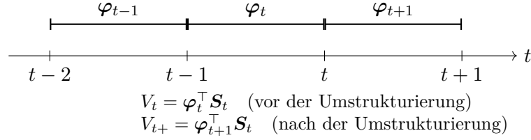
Abbildung 9.1.: Das Portfolio \varphi_t wird zum Zeitpunkt t - 1 auf Basis der Information \mathcal{F}_{t-1} gewählt und in [t-1, t) gehalten. Zum Zeitpunkt t wird zu \varphi_{t+1} umgeschichtet; V_t und V_{t+} sind die Vermögenswerte vor und nach der Umstrukturierung.
