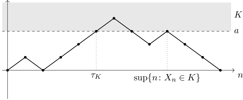
Abbildung 6.1.: Kontaktzeit \tau_K eines Pfades mit K = [a, \infty) : Ob \tau_K \leq n gilt, lässt sich am Pfad bis zur Zeit n ablesen. Für den letzten Aufenthalt in K ist das nicht der Fall: Erst die Zukunft entscheidet, ob der Pfad noch einmal nach K zurückkehrt.
