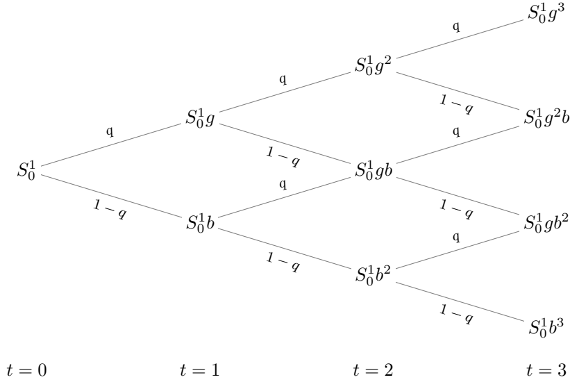
Abbildungung 9.2.: Kursverlauf S_t^1 der Aktie im CRR-Modell für T = 3 , mit den Abkürzungen g := 1 + r_g und b := 1 + r_b . Der Baum ist rekombinierend: S_t^1 hängt nur von der Anzahl D_t der Aufwärtsschritte ab. An den Kanten stehen die Übergangswahrscheinlichkeiten unter dem ÄMM Q aus Satz 9.20.
