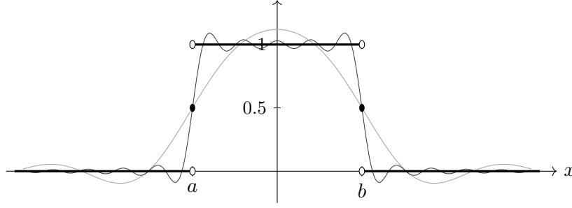
Abbildung 1.2.: Die Funktion x \mapsto (1/(2\pi))(R(x-a, T) - R(x-b, T)) für a = -1 , b = 1 und T = 4 (hellgrau), T = 15 (dunkelgrau) sowie ihr Grenzwert für T \rightarrow \infty (schwarz). Der Wert 1/2 an den Randpunkten erklärt den Term (1/2)\mathbb{P}(X \in \{a, b\}) in (1.24).
