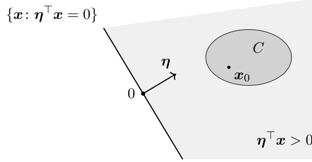
Abbildung 8.2.: Trennungssatz: Die konvexe Menge C mit 0 \notin C liegt im Halbraum \{\eta^\top x \geq 0\} , und mindestens ein Punkt x_0 \in C liegt nicht auf der trennenden Hyperebene.
