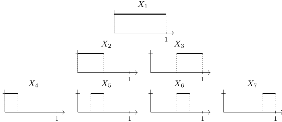
Abbildung 2.1.: Die wandernden Indikatoren X_1, \dots, X_7 auf [0, 1] . Die Träger werden immer kleiner (Konvergenz nach Wahrscheinlichkeit gegen 0), überstreichen aber in jeder Zeile ganz [0, 1] (keine f.s. Konvergenz).
