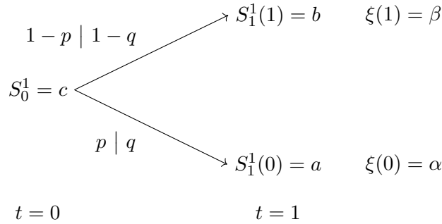
Abbildung 8.3.: Das Einperiodenmodell mit zwei Zuständen aus Beispiel 8.15. An den Kanten stehen die Wahrscheinlichkeiten unter \mathbb{P} und unter dem äquivalenten Martingalmaß \mathbb{Q} .
