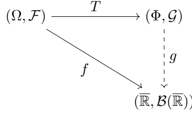
Abbildung 5.2.: Das Faktorisierungslemma: Eine \sigma(T) -messbare Abbildung f faktorisiert über T .
