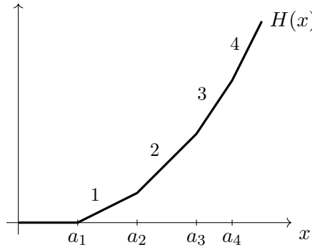
Abbildung 6.3.: Die Funktion H(x) = \sum_n (x - a_n)^+ aus dem Beweis von Satz 6.15 (vertikal gestaucht): Sie ist stückweise linear, und an jeder Stelle a_n wächst die Steigung um 1 (Zahlen an den Segmenten). Deshalb ist H konvex und H(x)/x \rightarrow \infty .
