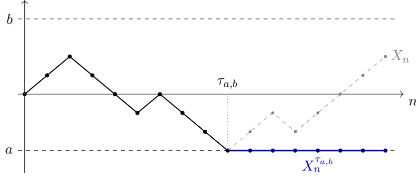
Abbildung 6.2.: Ein Pfad der einfachen Irrfahrt, der den Streifen zwischen a und b in a verlässt. Ab \tau_{a,b} bleibt der gestoppte Pfad X_n^{\tau_{a,b}} = X_{\tau_{a,b} \wedge n} konstant (blau), während X_n weiterläuft (grau gestrichelt). Insbesondere gilt |X_n^{\tau_{a,b}}| \leq b - a .
