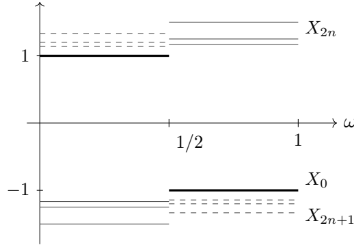
Abbildung 2.3.: Die Zufallsvariablen aus Beispiel 2.22: X_{2n} (durchgezogen, grau), X_{2n+1} (gestrichelt) für n = 1, 2, 3 und X_0 (schwarz). Die Werte springen zwischen den beiden Hälften von [0, 1] hin und her, die Verteilungen konvergieren aber gegen (1/2)(\delta_1 + \delta_{-1}) .
