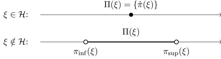
Abbildung 8.5.: Die Menge der arbitragefreien Preise nach Satz 8.26: ein Punkt für replizierbare Kontrakte, ein offenes Intervall sonst.
