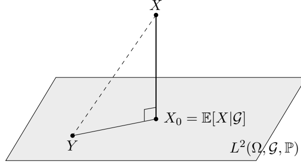
Abbildung 5.4.: Die bedingte Erwartung \mathbb{E}[X|\mathcal{G}] als orthogonale Projektion von X auf den Unterraum der \mathcal{G} -messbaren quadratintegrierbaren Zufallsvariablen. Für jedes andere \mathcal{G} -messbare Y gilt nach Pythagoras \mathbb{E}[(X - Y)^2] = \mathbb{E}[(X - X_0)^2] + \mathbb{E}[(Y - X_0)^2] .
